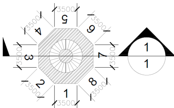
پلان قاعده ای منار جام در ولایت غور
