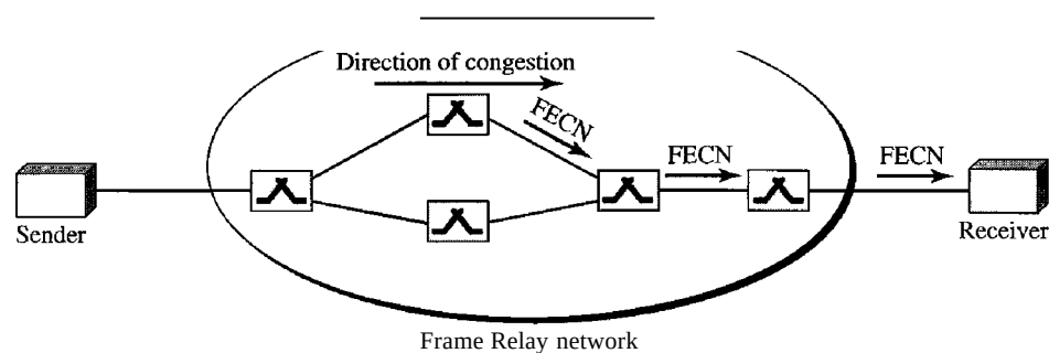
Figure 24.13 FECN
