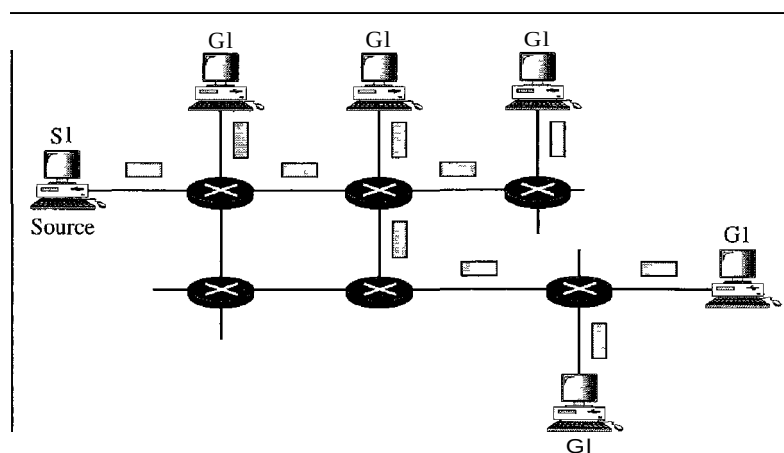
a. Multicasting
