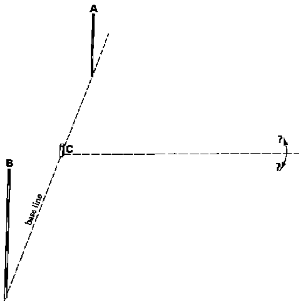
شکل ۲۱ الف. د قائمه زاویې جوړول ، لومړی مرحله Step 1 Fig. 21a Setting out a right angle, Step 1
