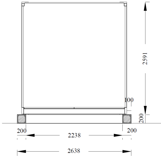
د کانتینر له پاره د کانکریت چوکاټ ۲۰۰ x ۲۰۰ ملی متر پرېک، نښه ۱:۳
