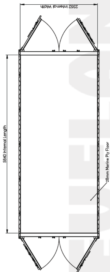
د ۲۰ فټه تونلي اوچت کانتینر پلان
