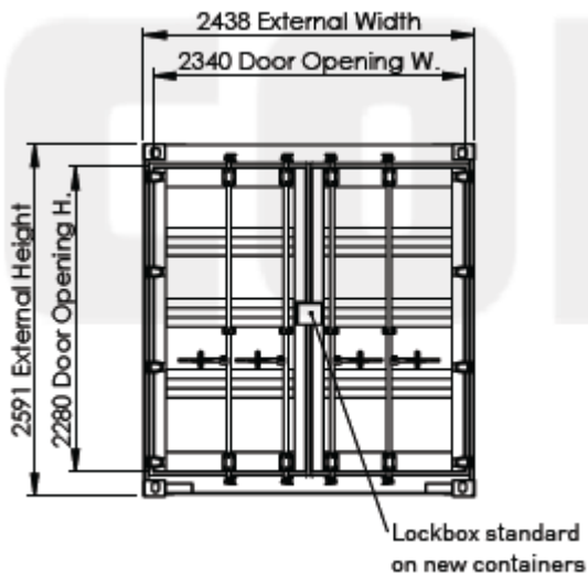
د ۴۵ فته سټنډرډ کانتینر دروازي لید
