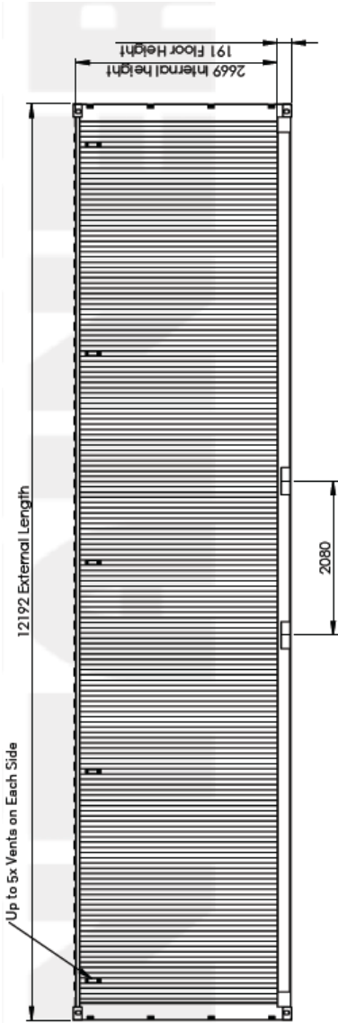
د ۴۰ فته تونلي اوچت كانتینر اوږد اړخ لید
