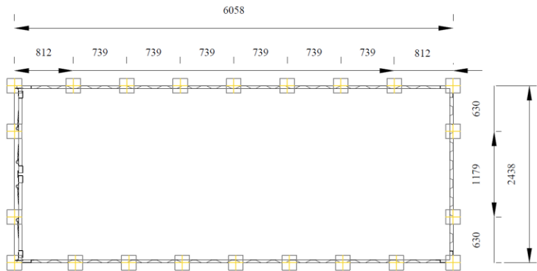
د کانکریت بلاک پلان ۲۰۰ x ۲۰۰ x ۲۰۰ ملی متر د ۲۰ فوټ کانتینر له پاره ، نښه ۱:۳
