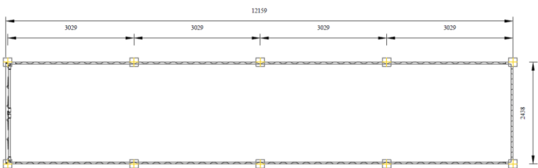
د کانکریت بلاک پلان ۲۰۰ x ۲۰۰ x ۲۰۰ ملی متر د ۴۰ فوټ کانتینر له پاره ، نښه ۱:۳
