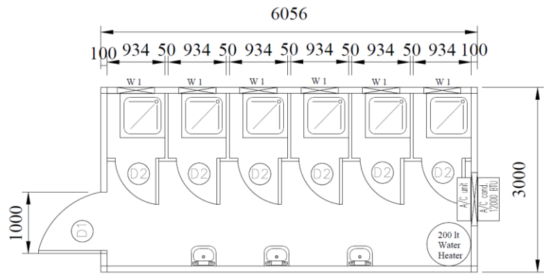
د تی آی ام د حمامونو لرونکي كانتینر فرنیچر پلان
