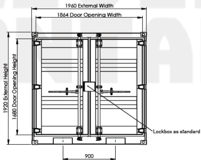
نمای دروازه کانتینر ۶ فوت حمل و نقل دریایی
