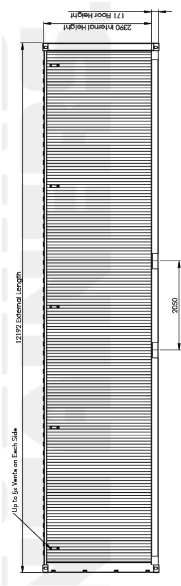
نمای جانبی کانتینر ۴۰ فوت استاندارد
