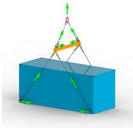
تصویری از شیوه بلند نمودن کانتینر ۲۰ فوت
