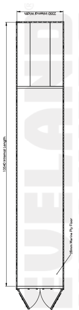
پلان کانتینر ۴۵ فوت بلند
