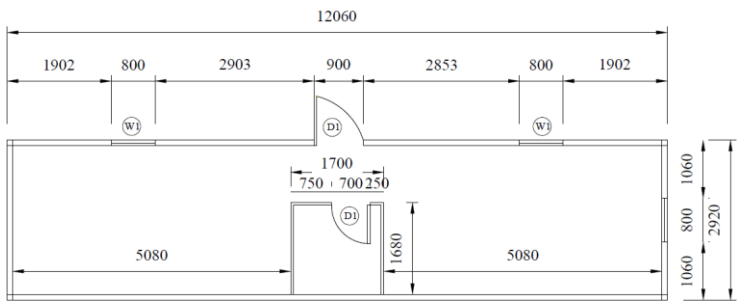
پلان کانتینر های تی آی ام
