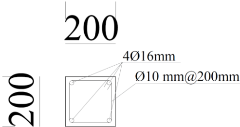
مقطع چوکات کانکریتی ۲۰۰ در ۲۰۰ ملی متر برای کانتینر ۴۰ فوت، مارک ۱:۳
