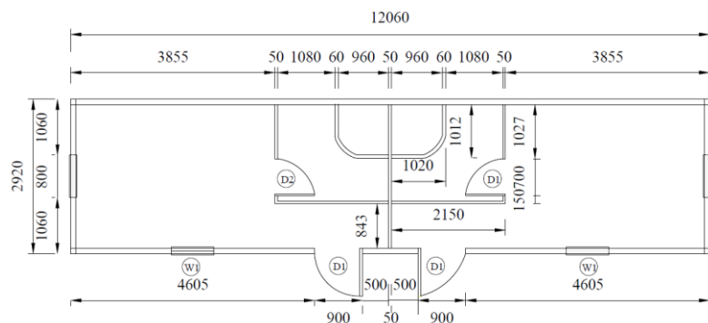
پلان کانتینر حمام دار تی آی ام
