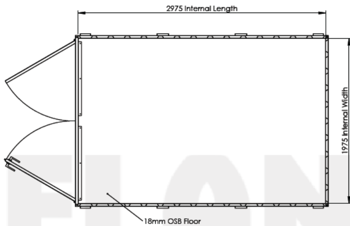
پلان کانتینر فلت پک ۳ در ۲ متر
