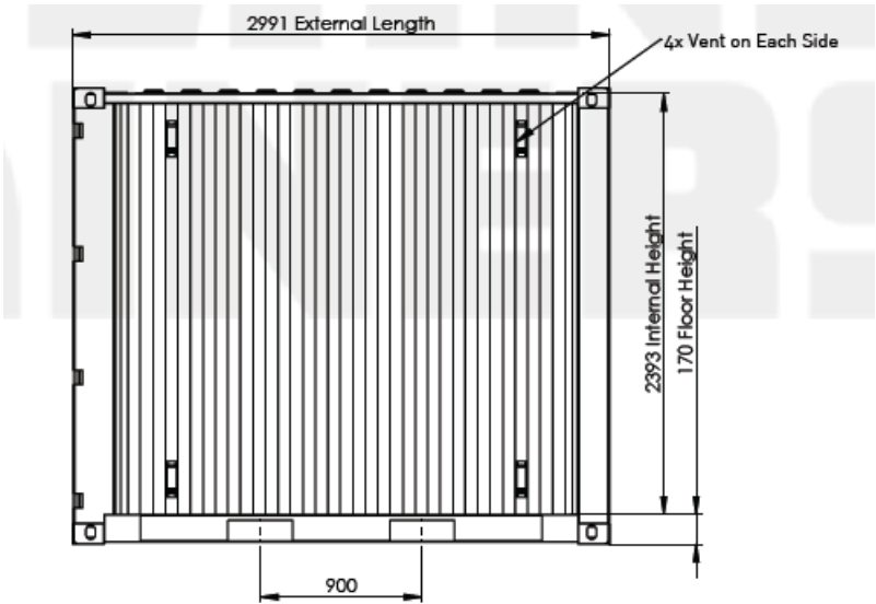
نمای جانبی کانتینر ۱۰ فوت مینی
