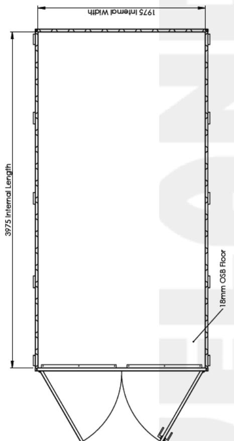
پلان کانتینر فلت پک ۴ در ۲ متر
