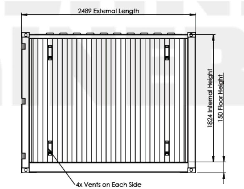
نمای جانبی کانتینر ۸ فوت مینی
