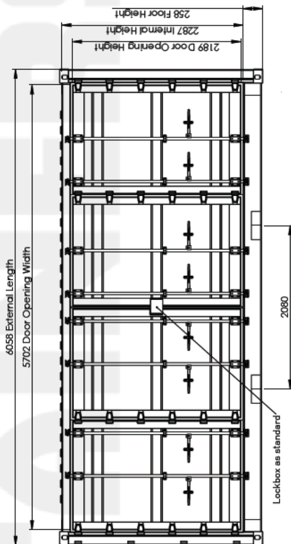
نمای جانبی کانتینر ۲۰ فوت استاندارد کنار باز شونده ۵۰۵۰
