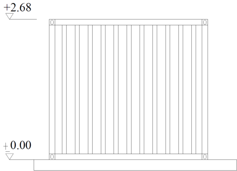
نمای پیشرو و عقب کانتینر تشناب دار تی آی ام
