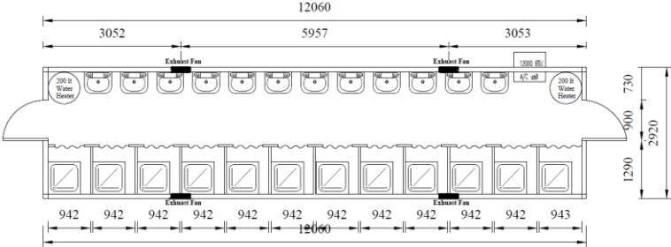
فرنیچر پلان کانتینر حمام تی آی ام
