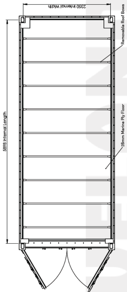
پلان کانتینر ۲۰ فوت ستندرد سر باز
