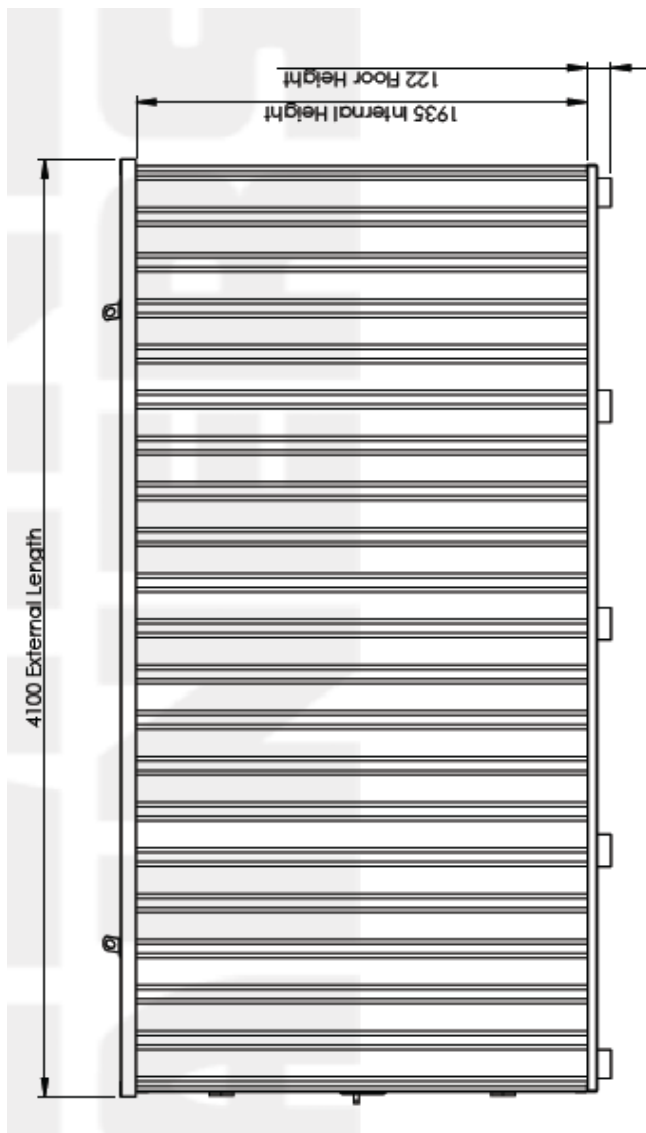
نمای جانبی کانتینر فلت پک ۴ در ۲ متر
