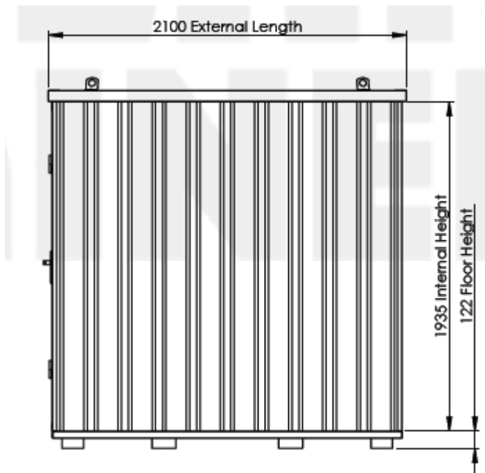
نمای جانبی کانتینر فلت یک ۲ در ۲ متر
