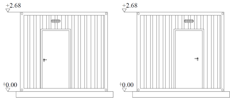
نما های پیشرو و عقب کانتینر حمام تونلی تی آی ام
