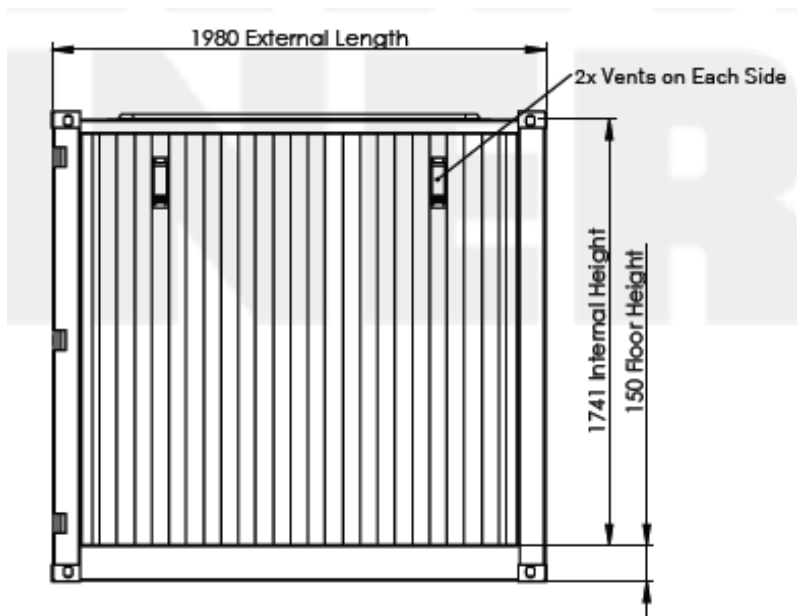
نمای جانبی کانتینر ۶ فوت حمل و نقل دریایی
