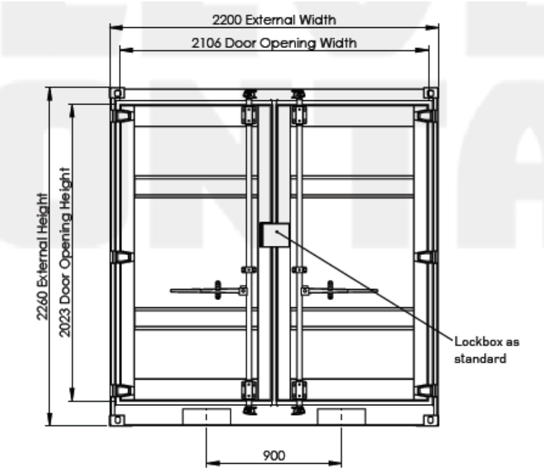
نمای دروازه کانتینر ۹ فوت مینی
