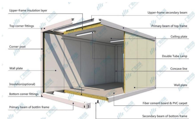
نمای سه بعدی تشریح کانتینر فلت پک
