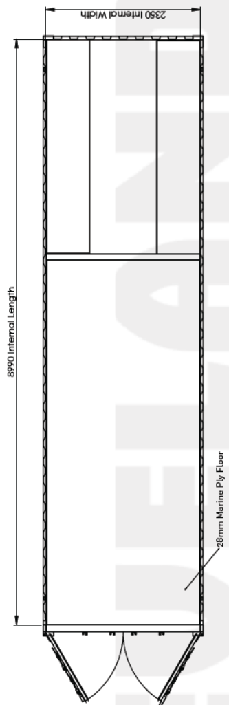
پلان کانتینر ۳۰ فوت
