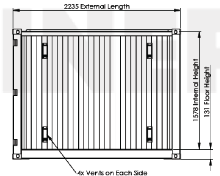
نمای جانبی کانتینر ۷ فوت مینی
