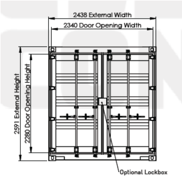
نمای دروازه کانتینر ۳۰ فوت
