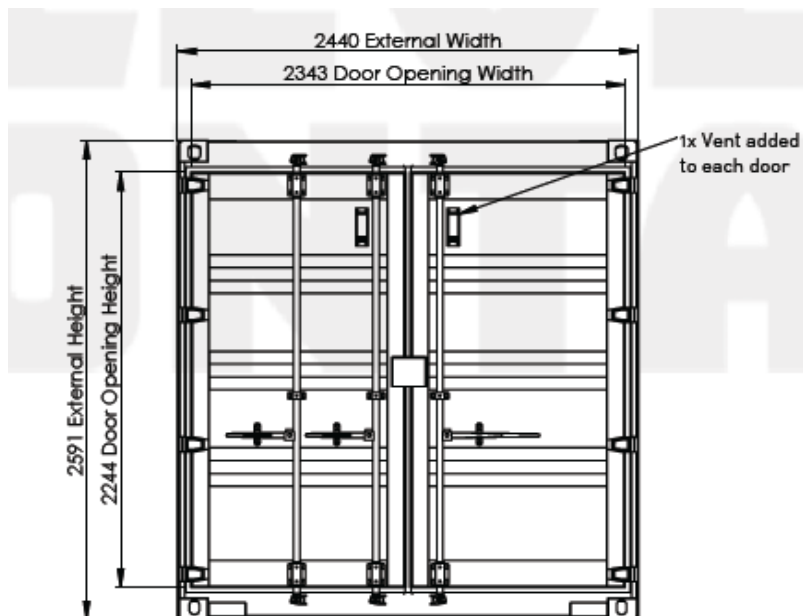
نمای دروازه کانتینر ۱۰ فوت دیو
