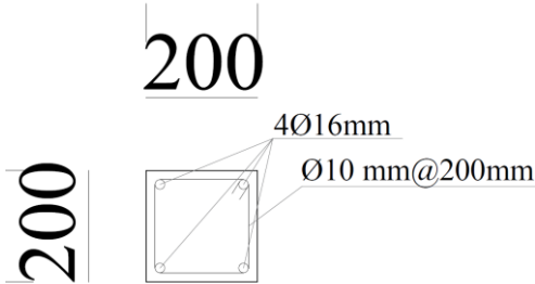
قطع چوکات کانکریتی ۲۰۰ در ۲۰۰ ملی متر برای کانتینر، مارک ۱:۳
