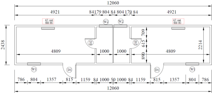
پلان کانتینر تشناب دار تی آی ام
