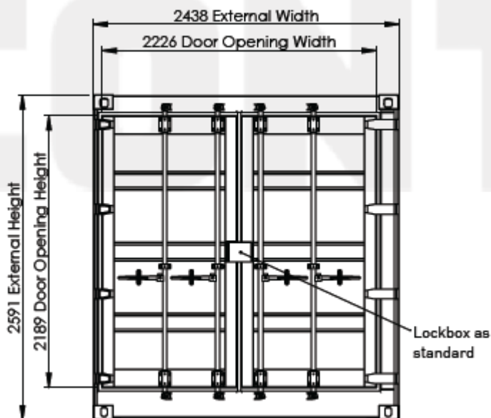
نمای دروازه کانتینر ۲۰ فوت استاندارد کنار باز شونده ۵۰۵۰
