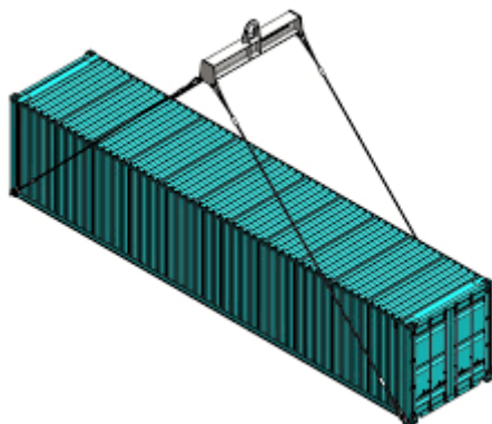
تصویری از شیوه بلند نمودن کانتینر ۴۰ فـت
