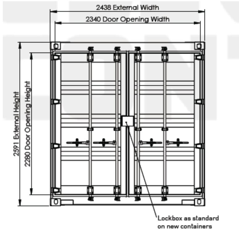
نمای دروازه کانتینر ۲۰ فوت استاندارد
