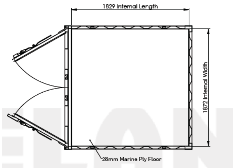
پلان کانتینر ۶ فت حمل و نقل دریایی
