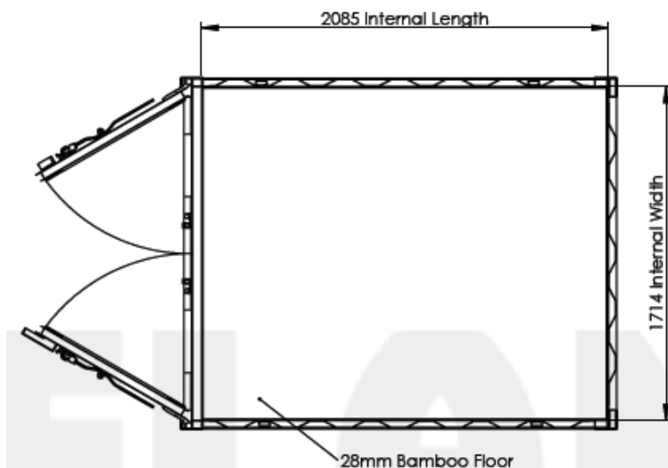
پلان کانتینر ۷ فوت مینی
