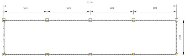
پلان بلوک کانکریتی ۲۰۰ در ۲۰۰ ملی متر برای کانتینر ۴۰ فوت، مارک ۱:۳
