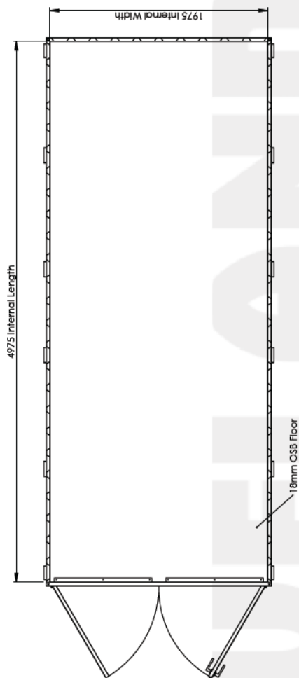
پلان کانتینر فلت پک ۵ در ۲ متر
