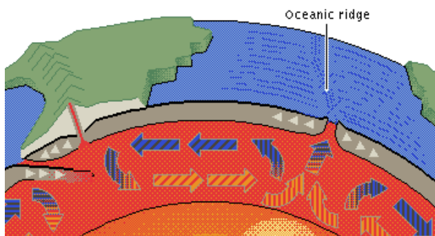
پروسه حرکت متداوم قشر زمین (Plate Tectonic)
