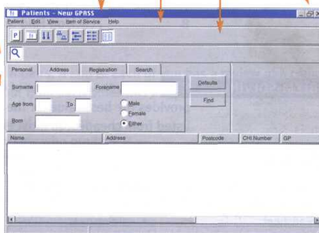
Fig 3 GPSS
