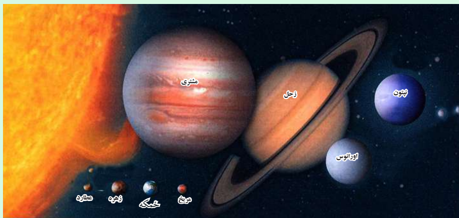
۱۱۸ - انځور: د پلوتو وړ ستوري په لرې واټن کې واقع دی.
