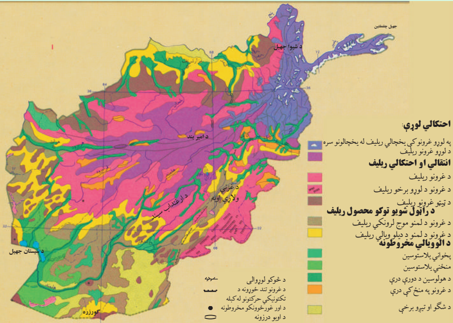
۱۱۰- انځور: د هېواد جيولوجيکي نقشه.
