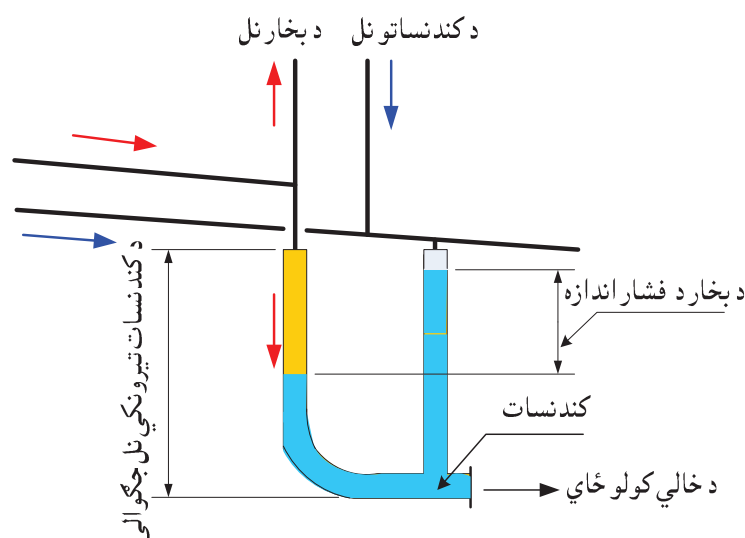
132- شکل د کندنسات تېروونکي نل جوړښت
