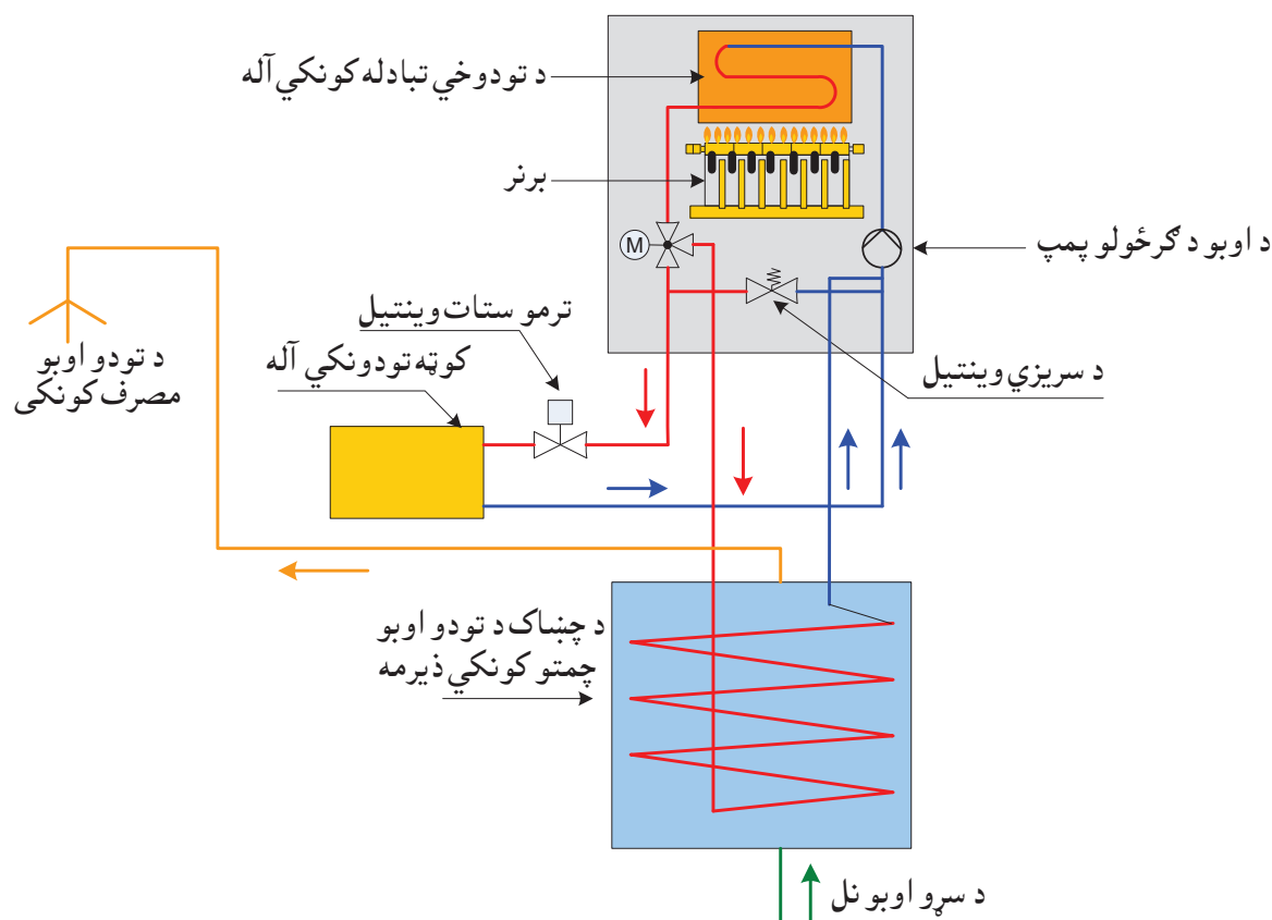
137- شکل په یوې جدا ذیرمې کې د تودو اوبو د چمتو کولو ځانګړتیاوي
