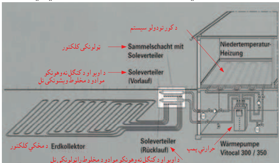
د مخکي د تودوخي څخه د ګټه اخستونکي یوه حرارتي پمپ شیمه (منبع: د فیسمن Viessmann د شرکت معلوماتي پاڼې)
