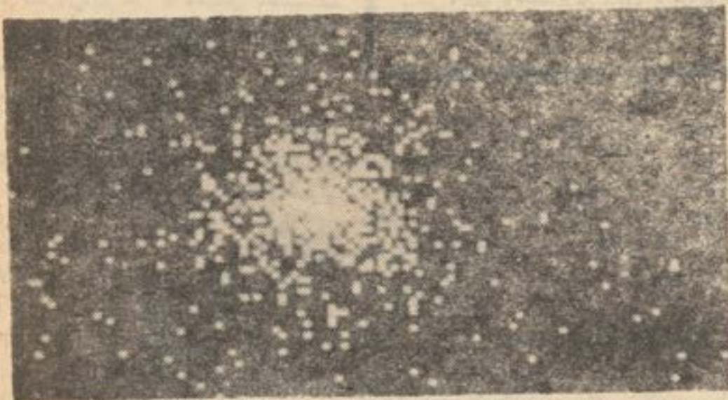
سینوس اکسل-۱ با فاصله ۶۰۰۰ سال نوری بعد بوده که در تصویر کامپیوتری ستاره ها دیده می شود
