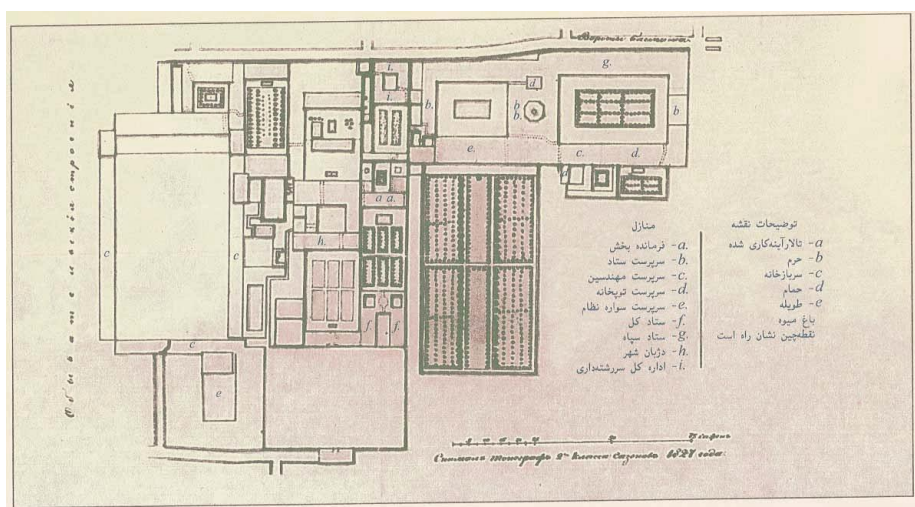
نقشه قصری متنسب به عباس میرزا که قرار بود در مجاورت تبریز بنا شود! (صفحه ۸)
